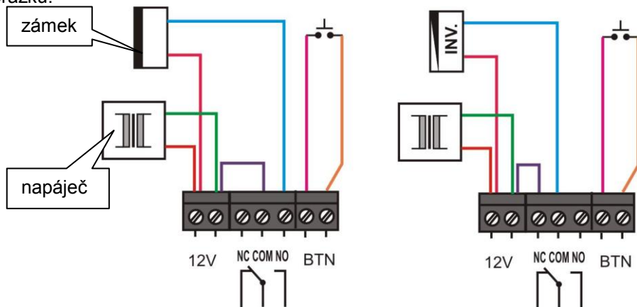
Připojení kabelů a zapojení standardního a inverzního zámku.
